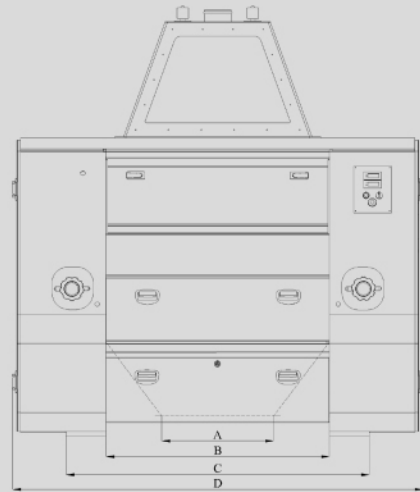
Tek Katli Vals / Single Storey Roller Mill / Одноэтажный Вальцевой Станок / Appareil A Cylindres Simple
