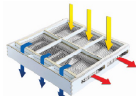
Elek Kasası (Geniş) Plansifter Frame (Large) Супер ситорама Boîte À Tamiser (Large)
