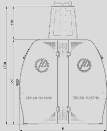
Tek Katli Vals / Single Storey Roller Mill / Одноэтажный Вальцевой Станок / Appareil A Cylindres Simple
