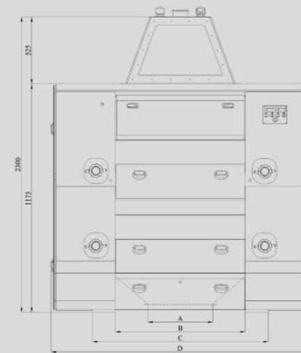
Çift Katli Vals / Double Storey Roller Mill / Двухэтажный Вальцевой Станок / Appareil A Cylindres Double
