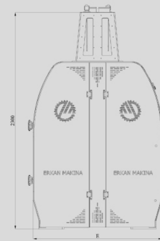
Çift Katli Vals / Double Storey Roller Mill / Двухэтажный Вальцевой Станок / Appareil A Cylindres Double
